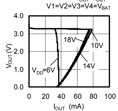
S-8243BAF
